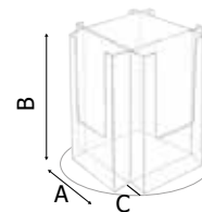
SLV15 DIMENSIONE INTERNA SCOMPARTI Larghezza: 111 mm Profondità: 28 mm
