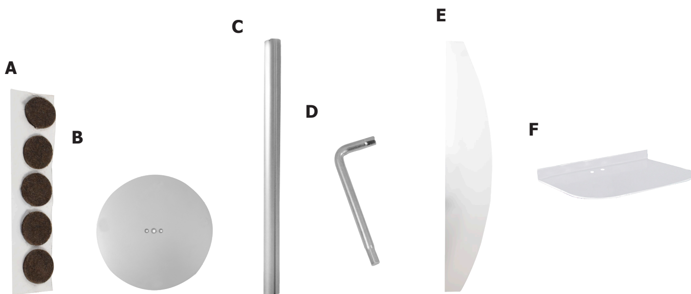
A feltrini per la base - B base in metallo - C montante in alluminio - D chiave a brugola - E vela - F ripiani sagomati (x4)
