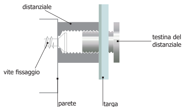
SCHEMA FISSAGGIO
