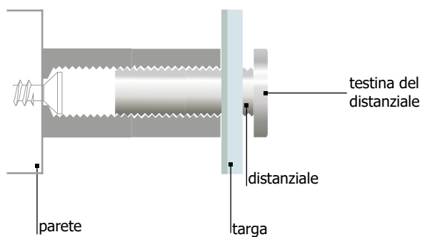
SCHEMA FISSAGGIO
