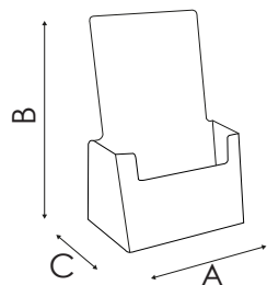
PDB102 DIMENSIONE INTERNA SCOMPARTI Larghezza: 110 mm Profondità: 32 mm
