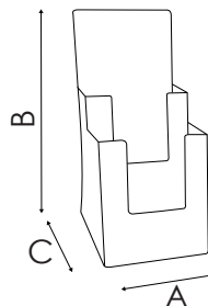
PDB202 DIMENSIONE INTERNA SCOMPARTI Larghezza: 110 mm Profondità: 32 mm
