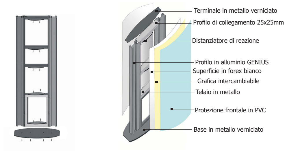
STRUTTURA INTERNA
